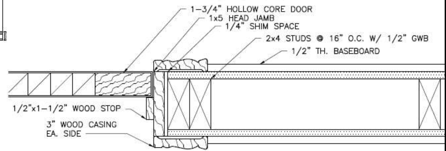
3 DOOR JAMB SECTION A1 SCALE: 3"=1'-0"
